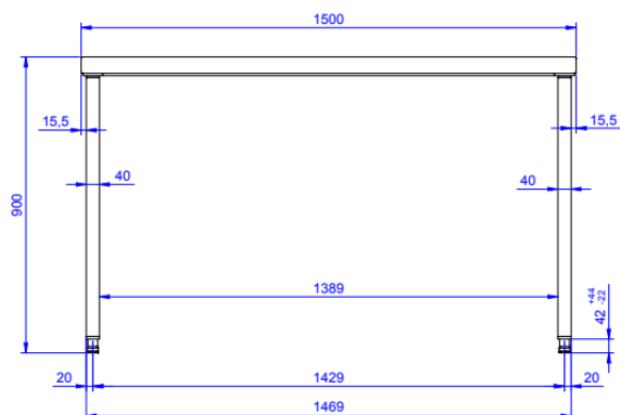
Edestä
